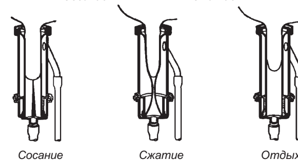
Рис. 2.13. Схема работы доильного стакана при разных способах доения.
